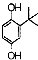
TBHQ
