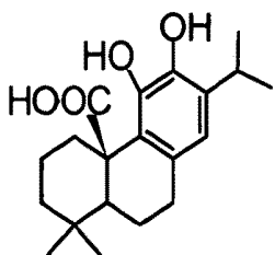
Carnosic acid
