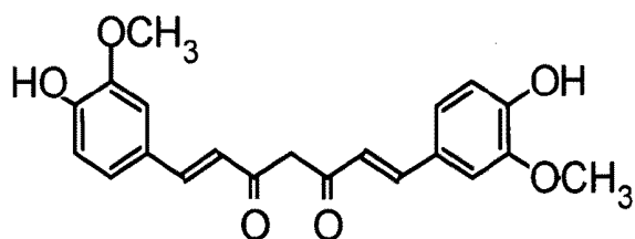
Curcumin
