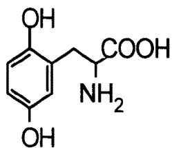
Para L-dopa
