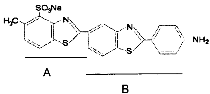
Primulin
