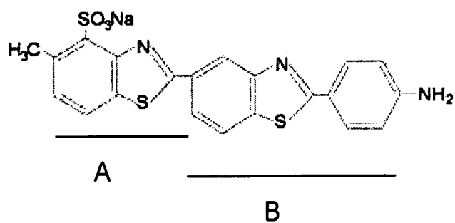
Primulin
