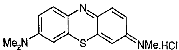
Azure B
