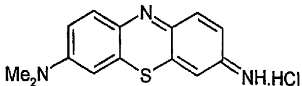
Azure A
