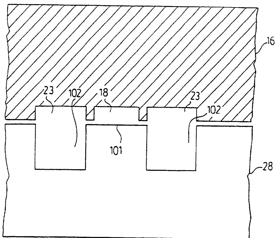
FIG. 22 c-c
