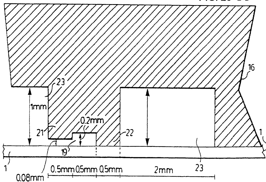
FIG. 23 D-D
