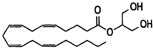
2-ARACHIDONYLGLYCEROL (2-AG)
