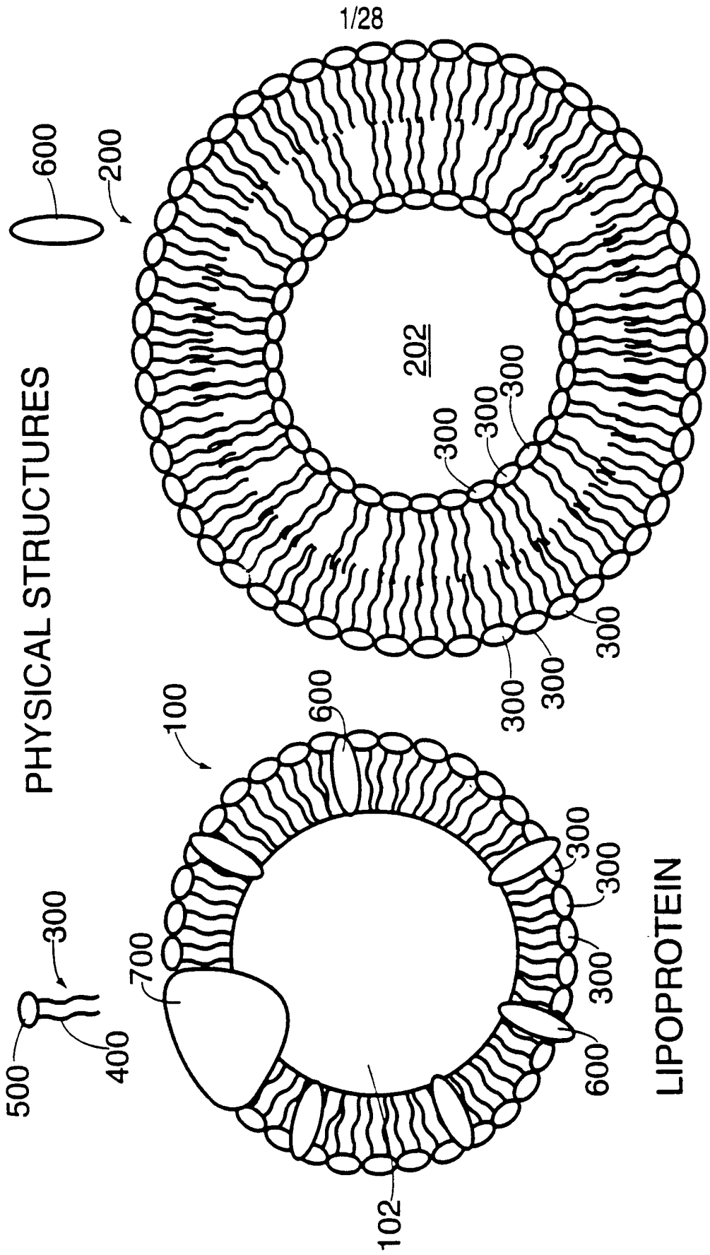
LIPOSOME
