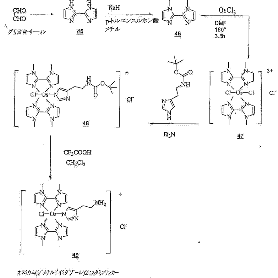
オスミウム(ジメチルピイミダゾール) 2 ヒスタミンリンカー(49)の合成
