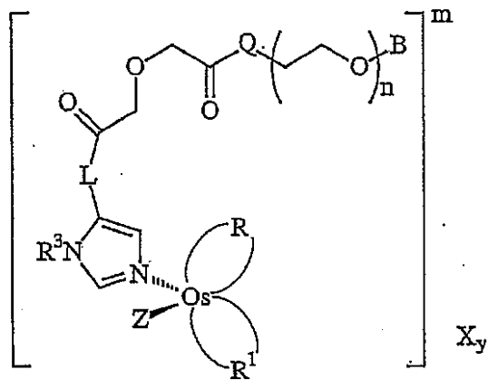
化合物 4
