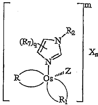
化合物 1
