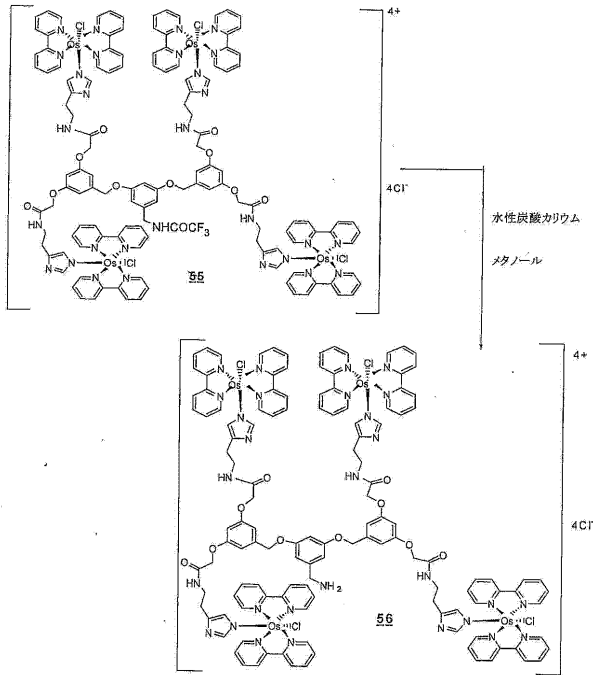
テトラオスミウムリンカー(56)の合成
