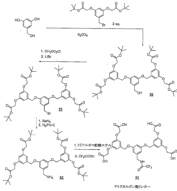
テトラカルボン酸リンカー(53)の合成
