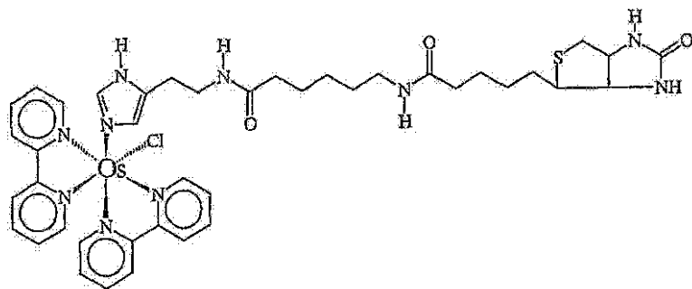
化合物 57
