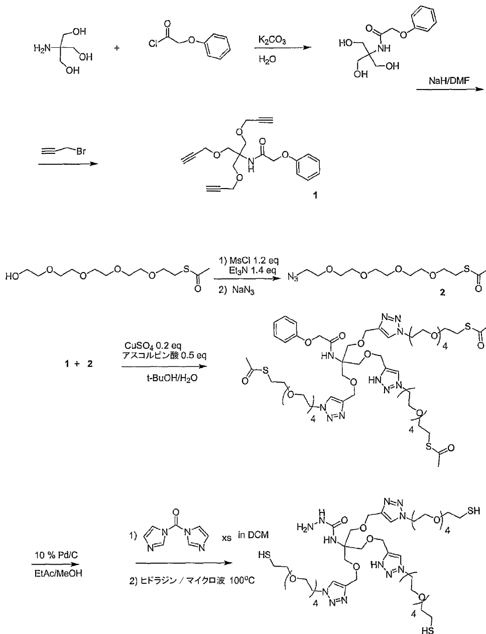
スキーム 18c
