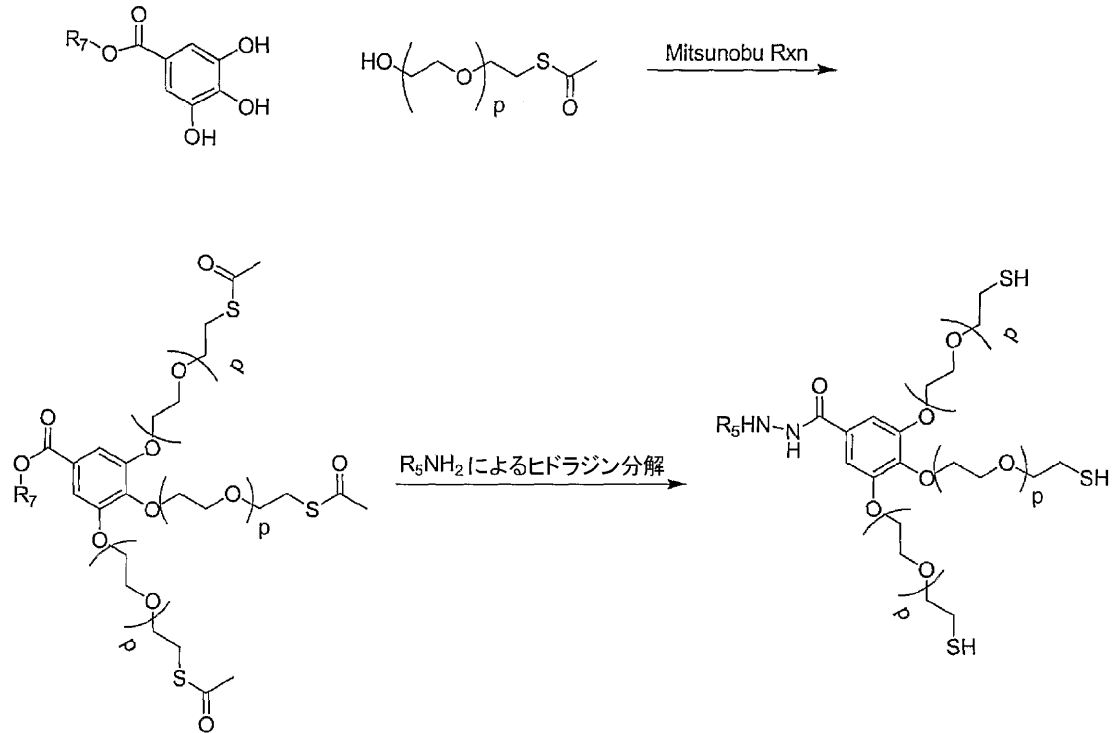
スキーム5c
