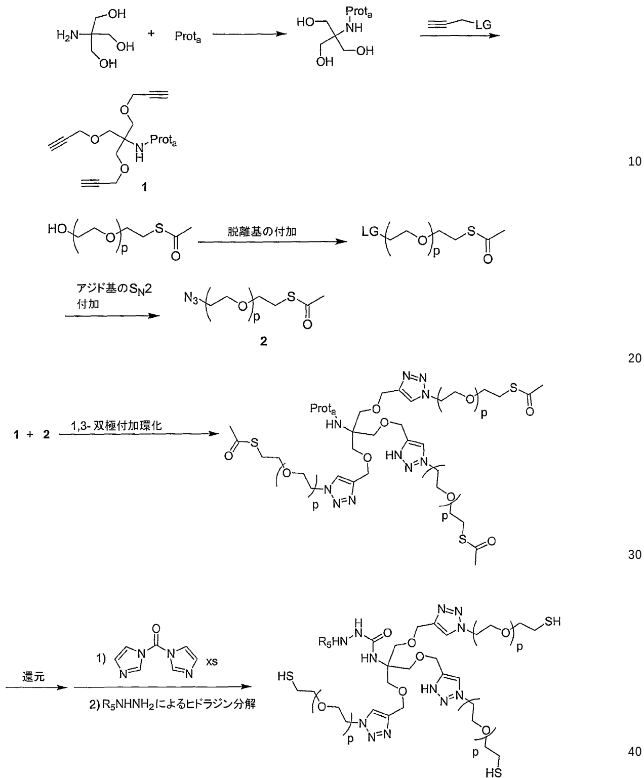
スキーム5b
