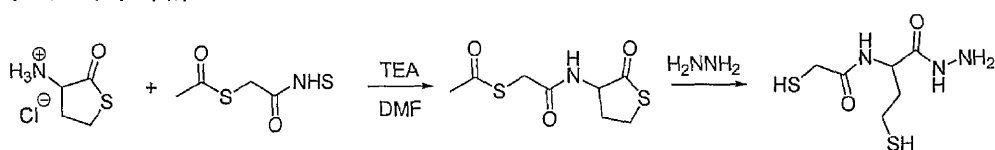
スキーム 17a
