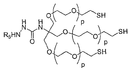
スキーム5a
