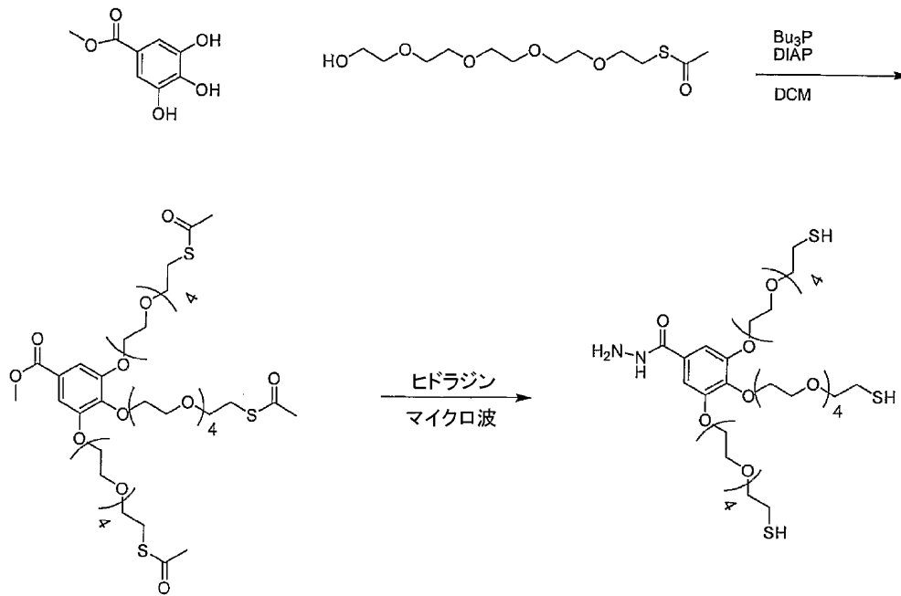
スキーム 18b
