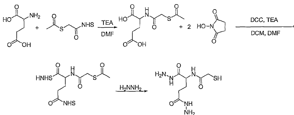
スキーム 17c
