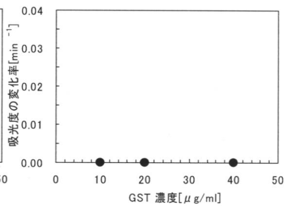
( f ) 疎水性プレート ( PBS+Tween20+BSA )
