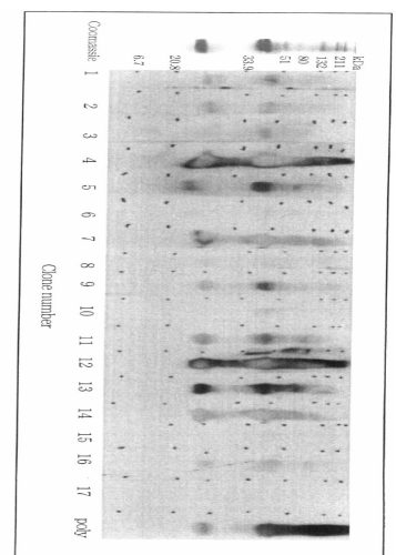
【図1】ラズベリーチンに結合する抗体の濃度 1-7はコントロール、8-17は抗NC1単クローナル抗体を示す
