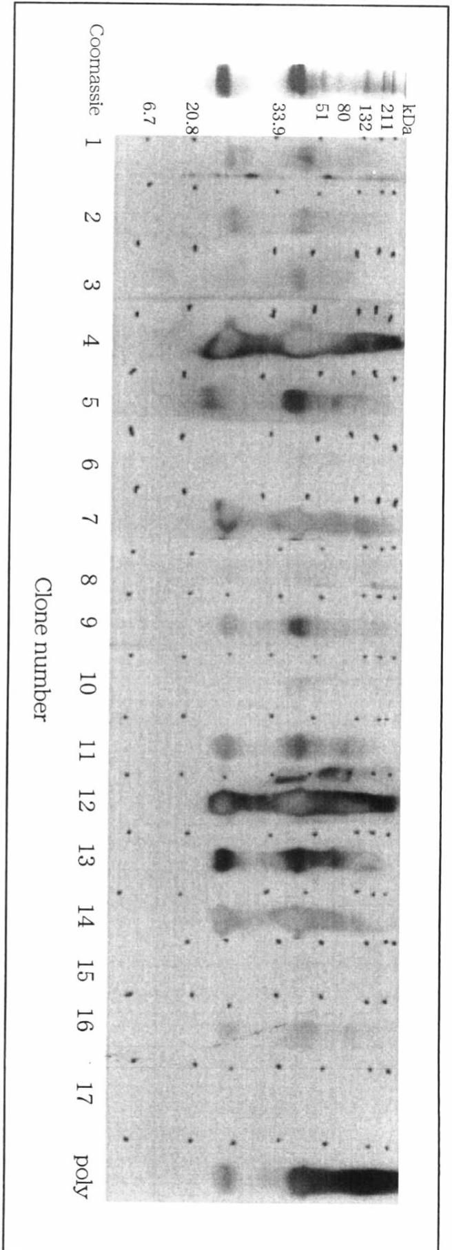
【図1】 ウエスタンブロッティングに依る抗体の選出
