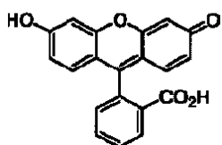
式B
