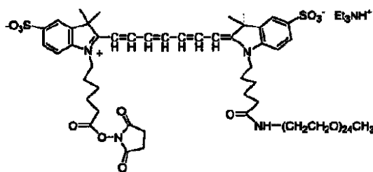
化合物 No. 61
