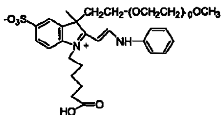
化合物 No. 69
