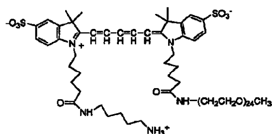
化合物 No. 88
