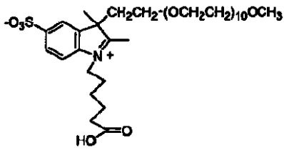
化合物 No. 31
