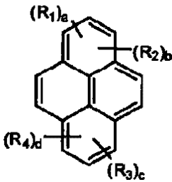
式 V
