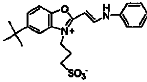
化合物 No. 50
