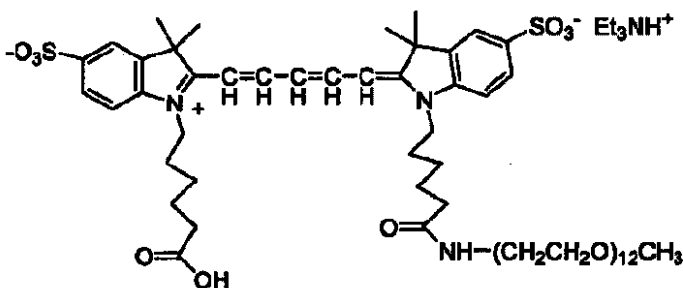
化合物 No. 8
