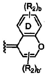
式 2
