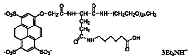
化合物 No. 82
