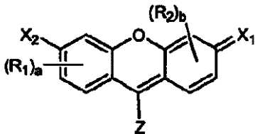
式III
