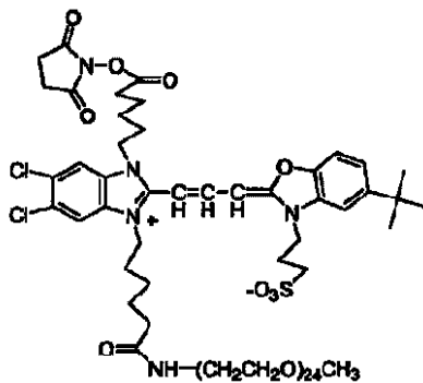
化合物 No. 52
