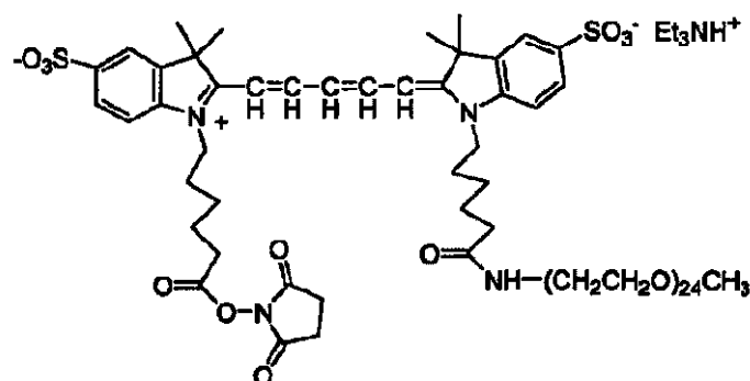
化合物 No. 7
