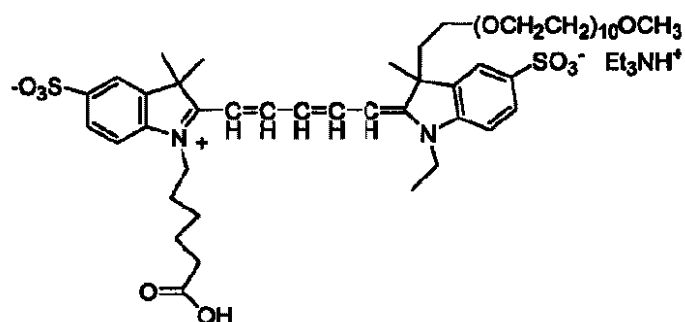
化合物 No. 30
