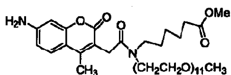
化合物 No. 90
