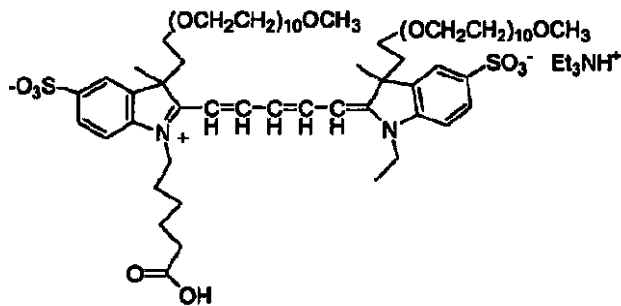
化合物 No. 35
