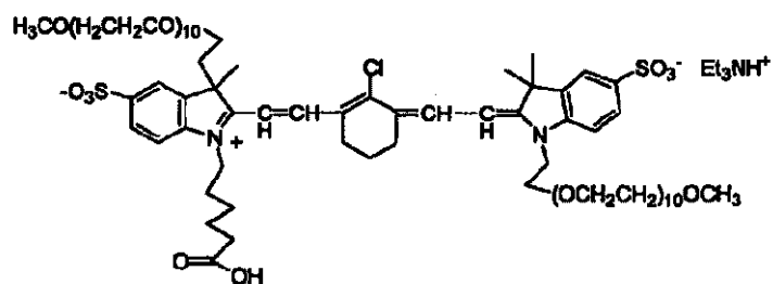
化合物 No. 72
