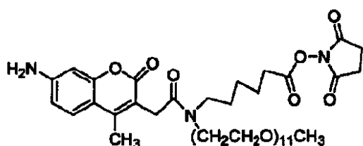
化合物 No. 92
