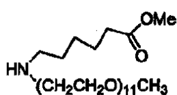
化合物 No. 89
