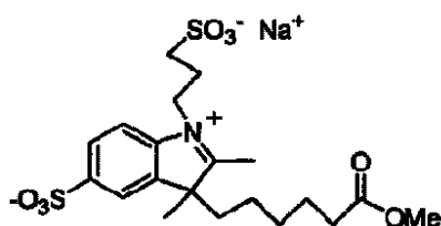
化合物 No. 14
