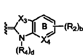
式1
