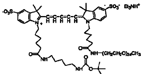
化合物 No. 87
