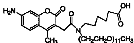
化合物 No. 91
