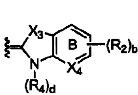
式 1
