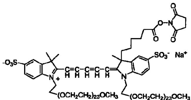
化合物 No. 41
