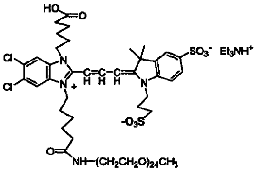
化合物 No. 55
