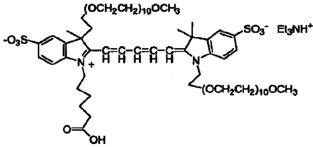
化合物 No. 37
