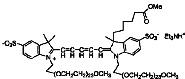
化合物 No. 40
