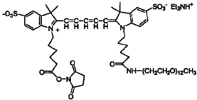
化合物 No. 9
