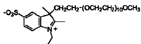
化合物 No. 29
