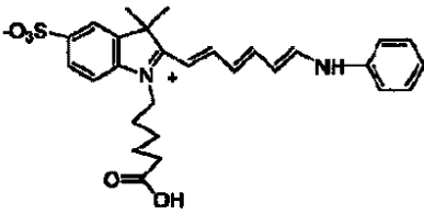
化合物 No. 59
