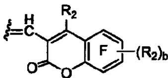
式 4
