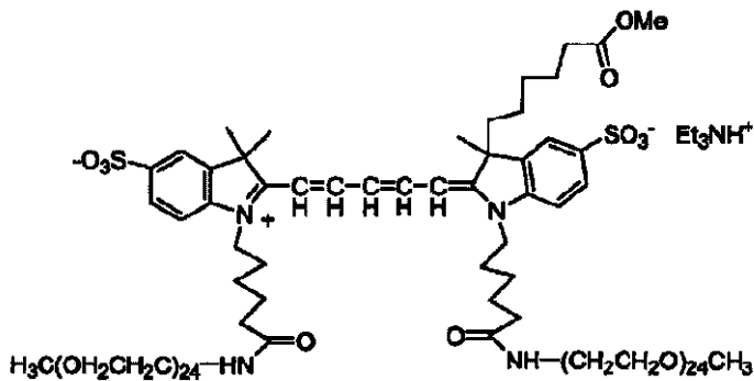
化合物 No. 21
