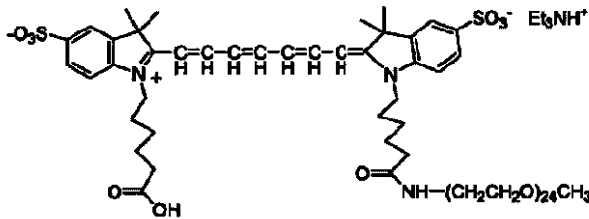
化合物 No. 60
