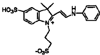
化合物 No. 54
