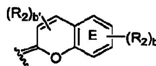
式3
