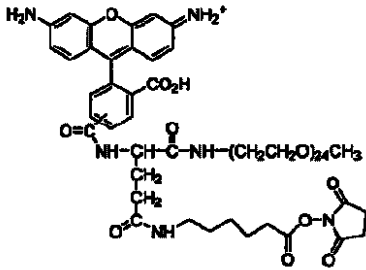
化合物 No. 77
