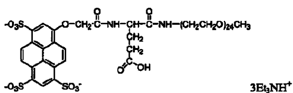
化合物 No. 81
