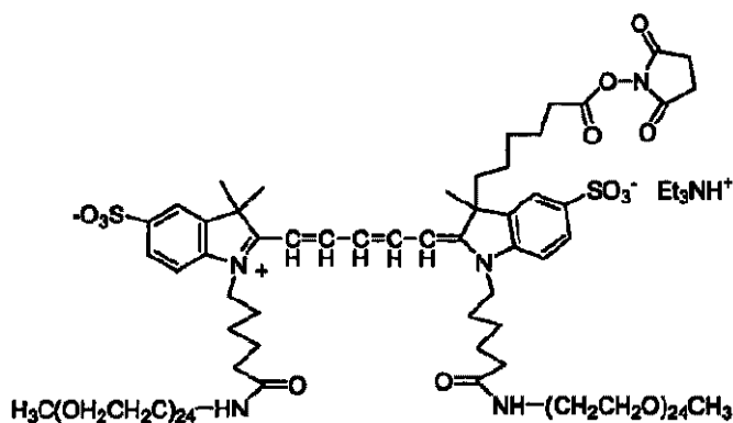
化合物 No. 23
