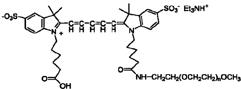
化合物 No. 11
