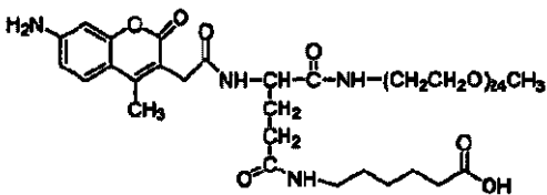
化合物 No. 79
