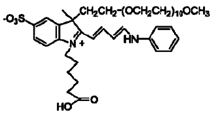
化合物 No. 32
