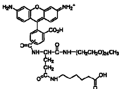
化合物 No. 76
