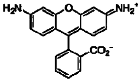
式C
