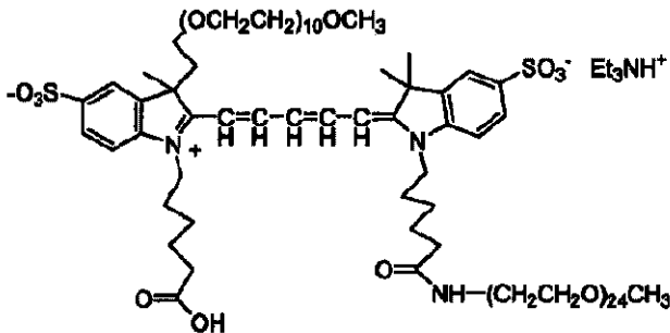
化合物 No. 33
