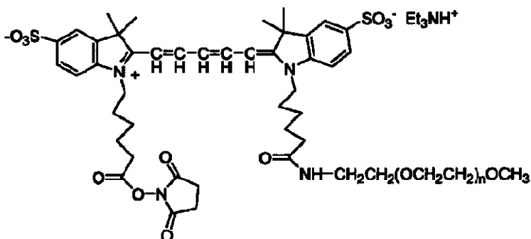
化合物 No. 12
