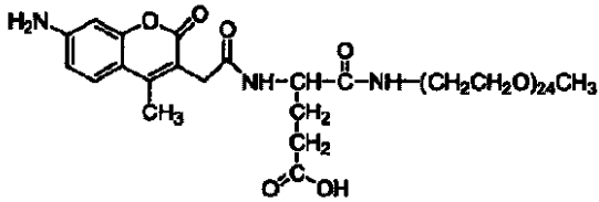
化合物 No. 78
