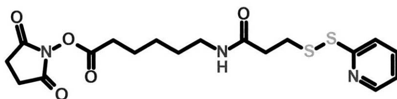
LC-SPDP スクシンイミジル 6-[3(2-ピリジルジチオール)プロピオンアミド]ヘキサノエート
