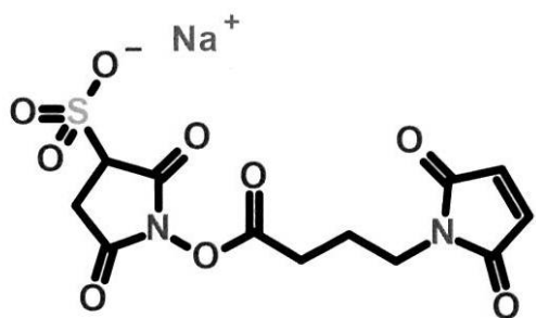
スルホ-GMBS(N- \gamma -マレイミドブチリル-オキシルホスクシンイミドエステル)
