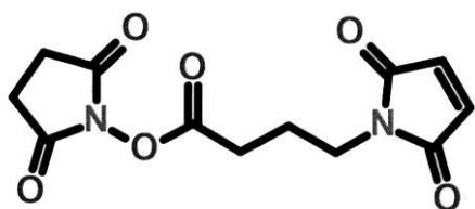
GMBS(N- \gamma -マレイミドブチリル-オキシスクシンイミドエステル)
