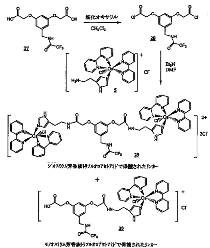
ジオスミウム芳香族トリフルオアセチドで保護されたリカー(29)及びモノスミウム芳香族トリフルオアセチドで保護されたリカー(30)の合成
