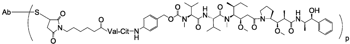
Ab-MC-vc-PAB-MMAE (vcMMAE)
