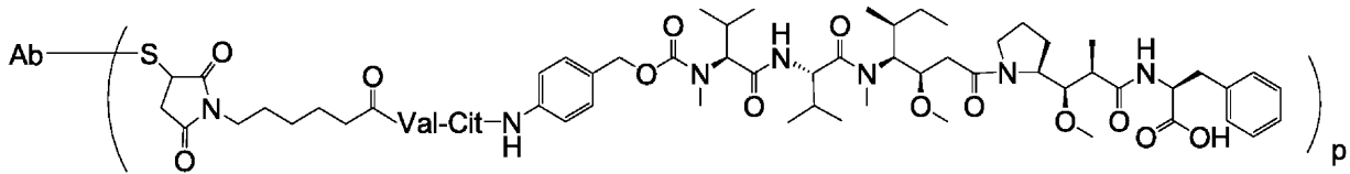
Ab-MC-vc-PAB-MMAF (vcMMAF)
