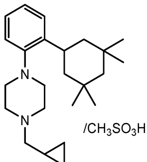
化合物 B
