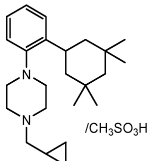
化合物 B
