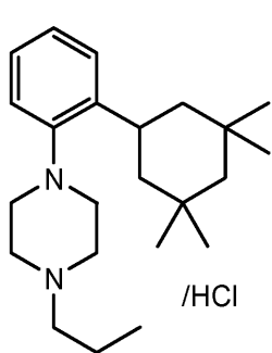
化合物 A
