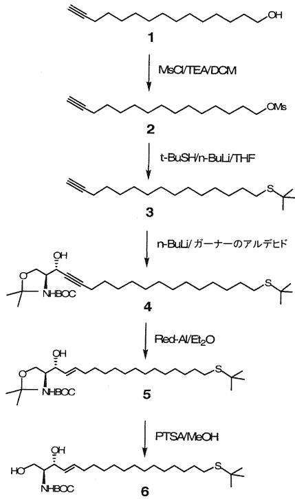
Figure 1a. 典型的なチオール化S1P関連抗原の合成
