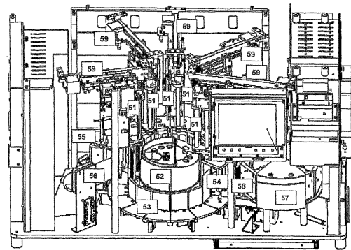
システム配置の正面図
