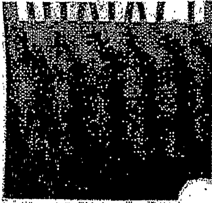
B. 16 mM tris 碱
