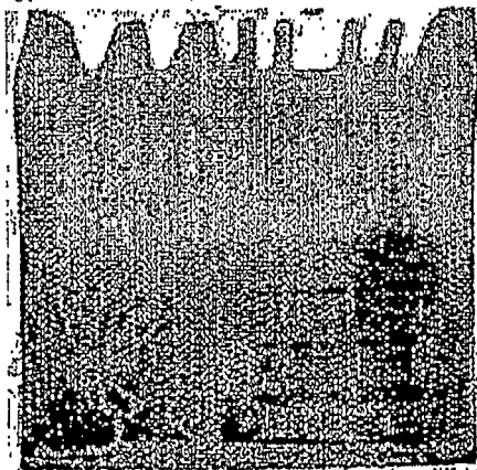
C. 16 mM 丁胺
