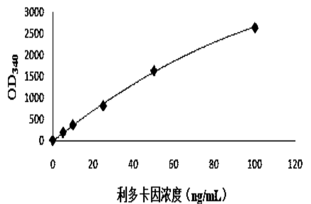
利多卡因校准曲线
