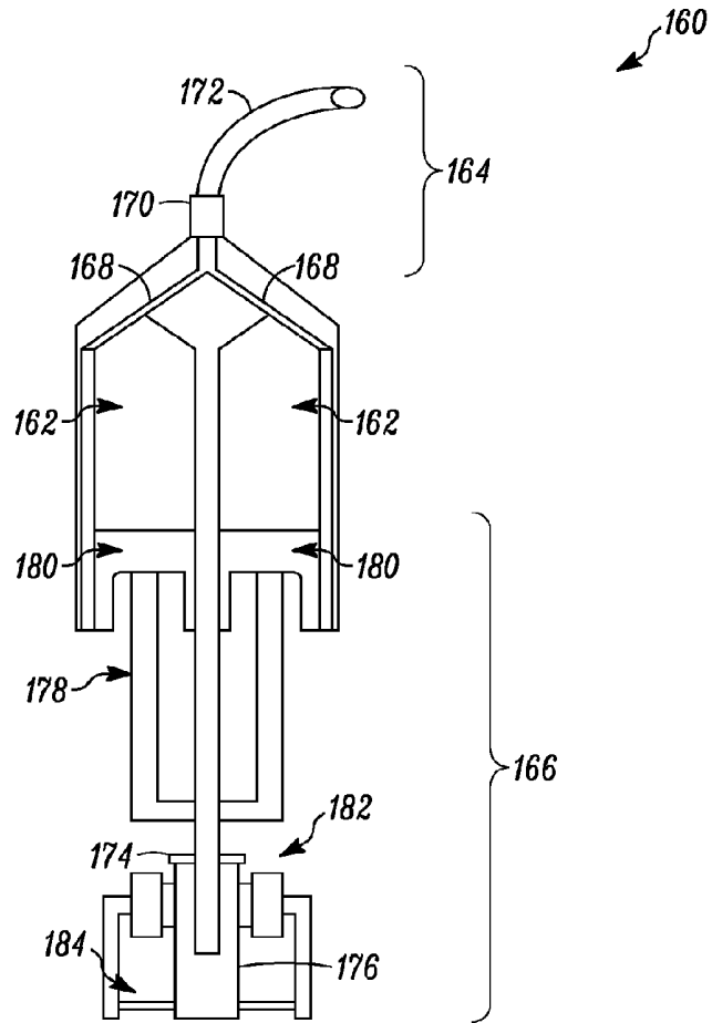
FIG. 11A
