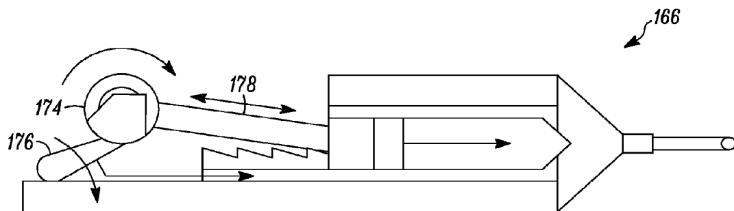
FIG. 11B
