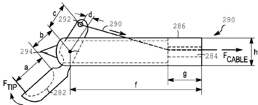
FIG. 17A
