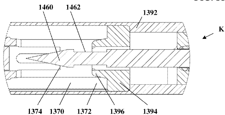
FIG. 10E
