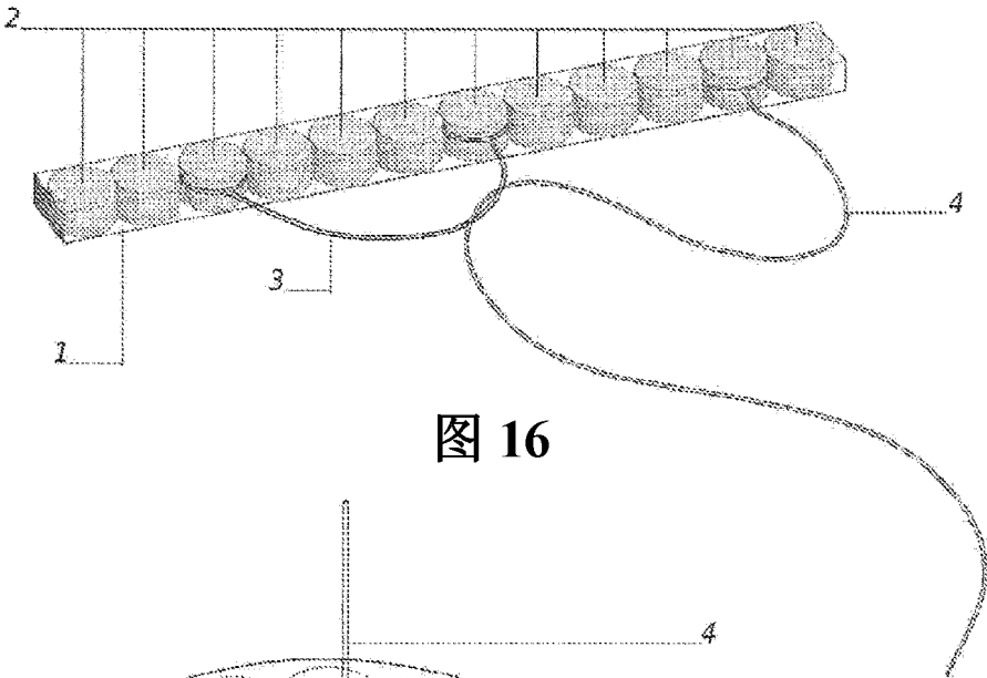
模块化磁吻合装置：实例 3
