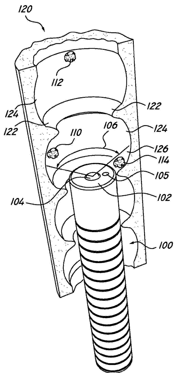
图 1 现有技术
