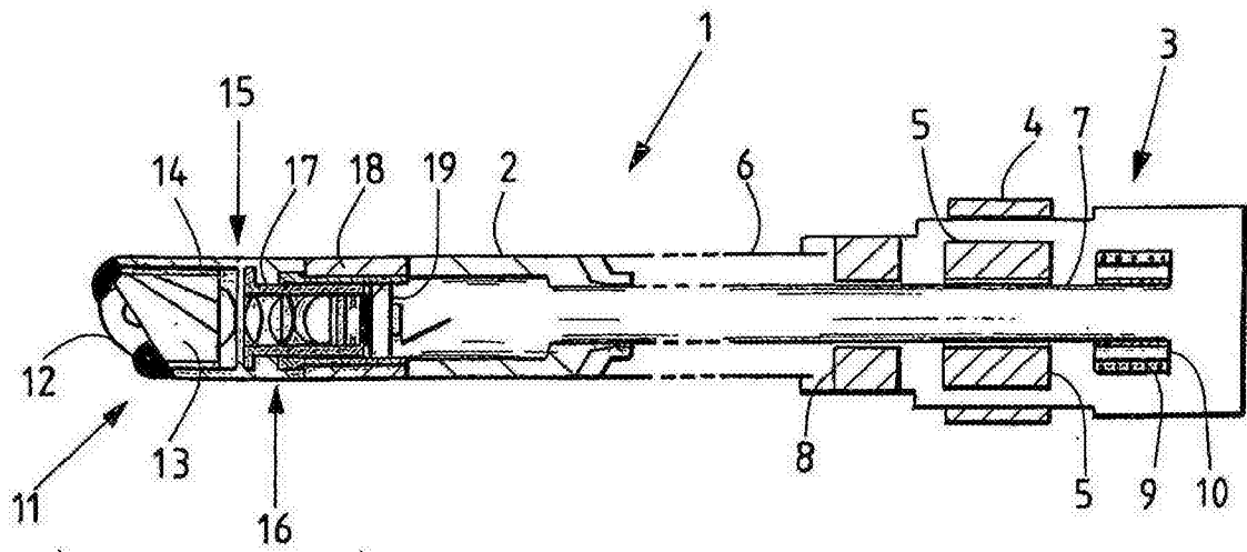
图 1(现有技术)
