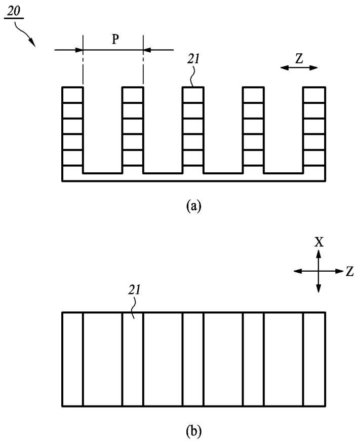
도면6
