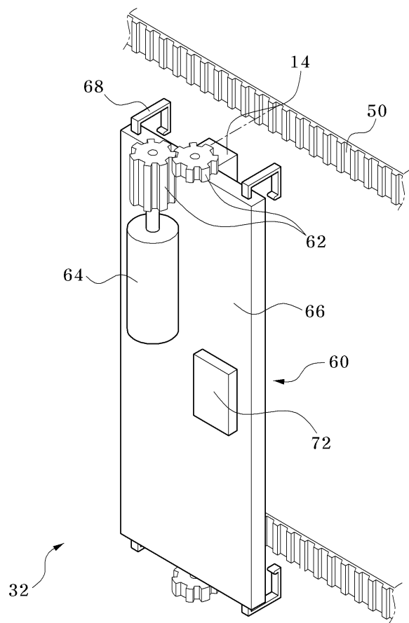
도면8
