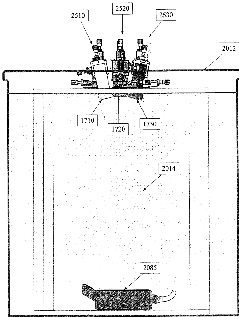
탱크내의 조립된 테스트 설비
