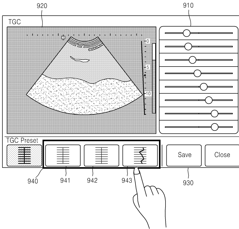
도면9c
