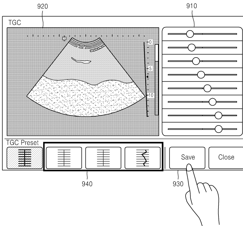
도면9a
