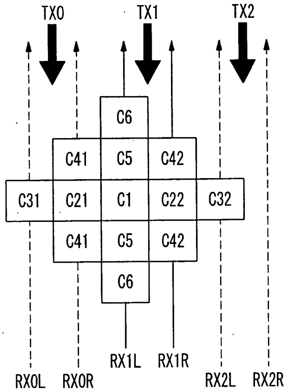
FIG. 5B
