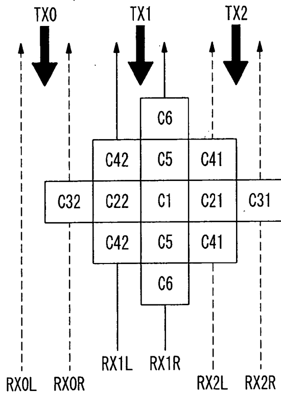
FIG. 5C
