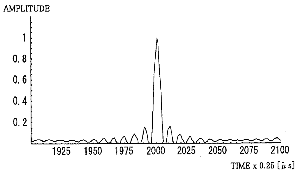
(a) NO DOPPLER SHIFT
