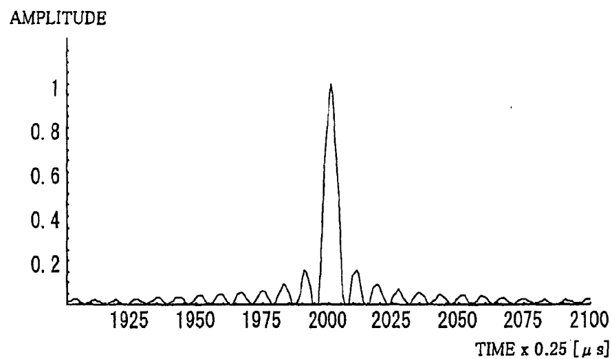
(a) NO DOPPLER SHIFT
