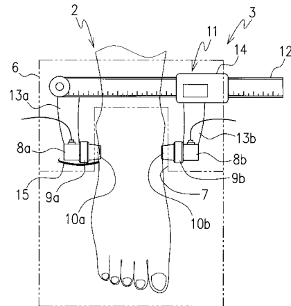
2…踵 3…測定部 8a,8b…超音波探触子 10a,10b…アタッチメント 11…デジタルキャリパ(踵幅測定手段) 15…熱電対(温度センサ)
