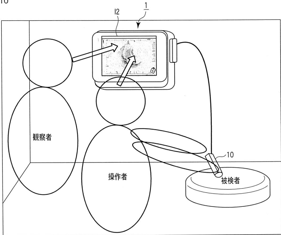
タブレットモード(操作者&観察者) 画像表示領域(超音波画像)12のみ表示
