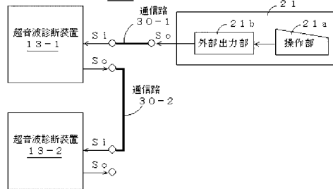
(図 10) 超音波診断装置システム 107
