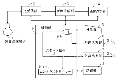
(図 12) 超音波診断装置 14
