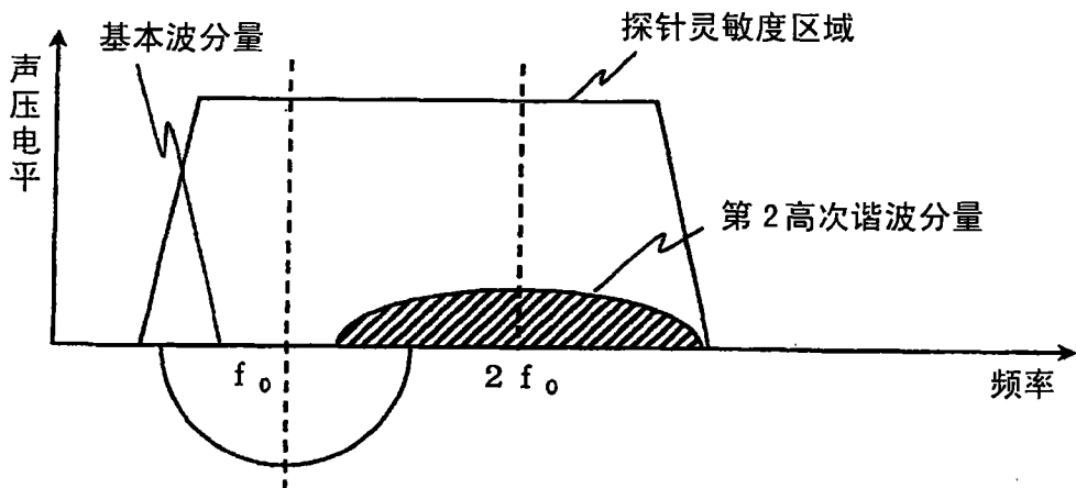
(b) 基于第2脉冲的反射回声分量
