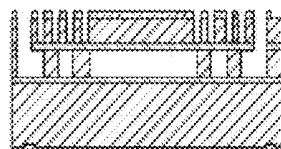
(F) DRIE etch top Si
