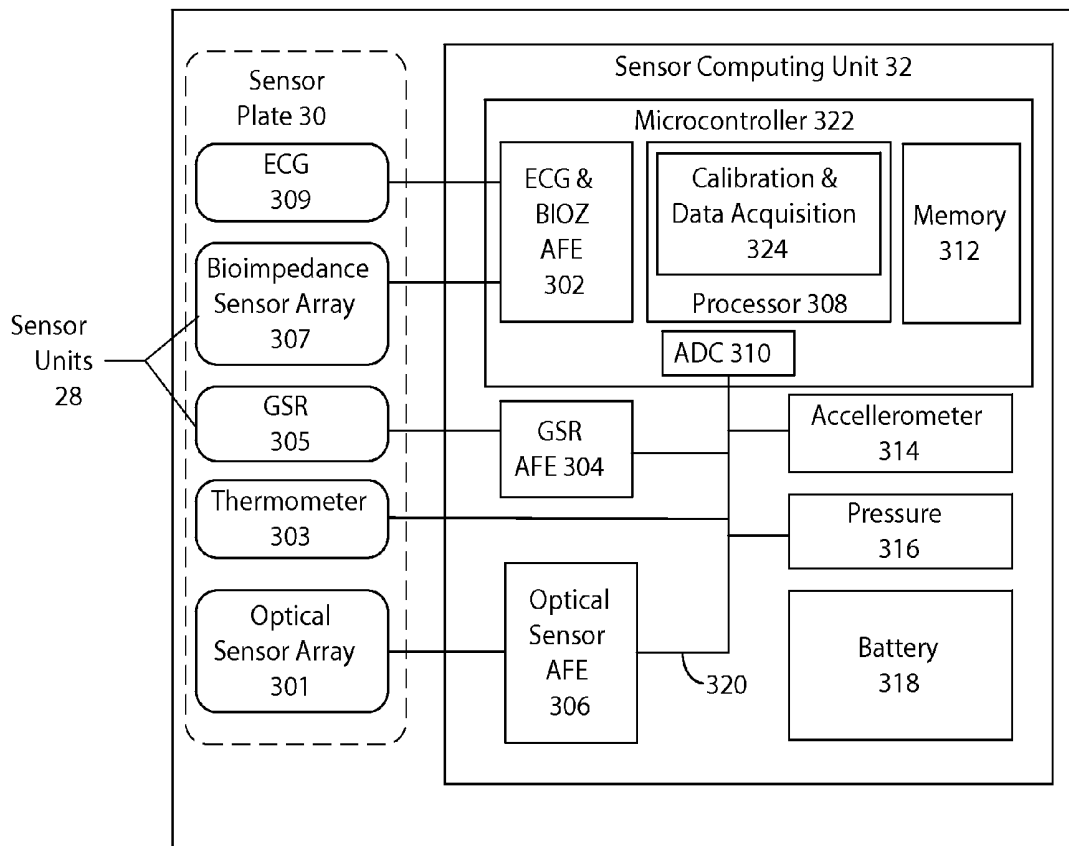
Sensor Module 10
