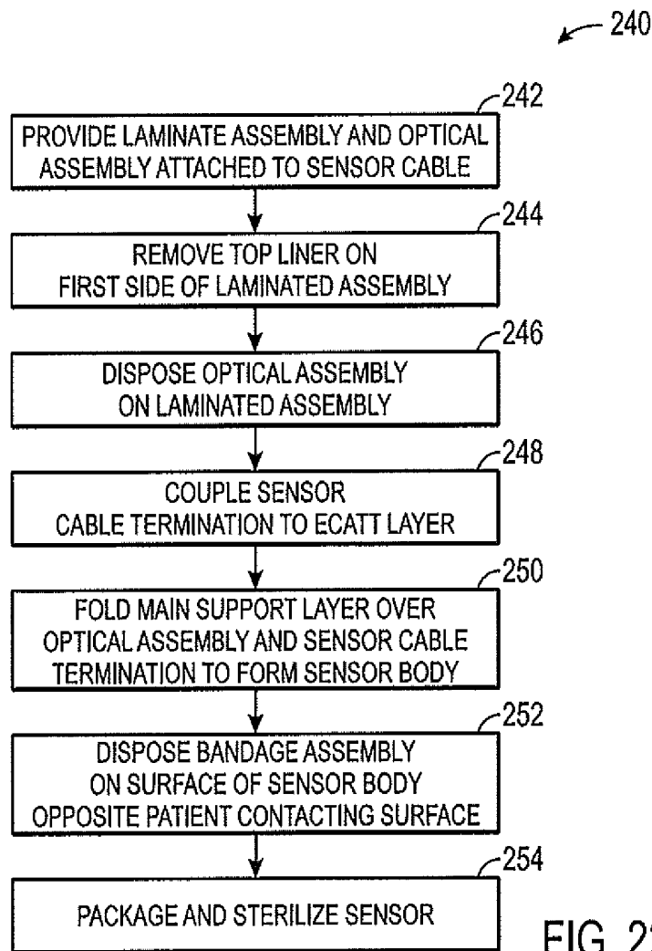
FIG. 21
