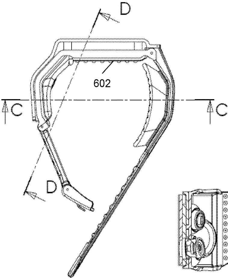
SCALE 1 : 1
