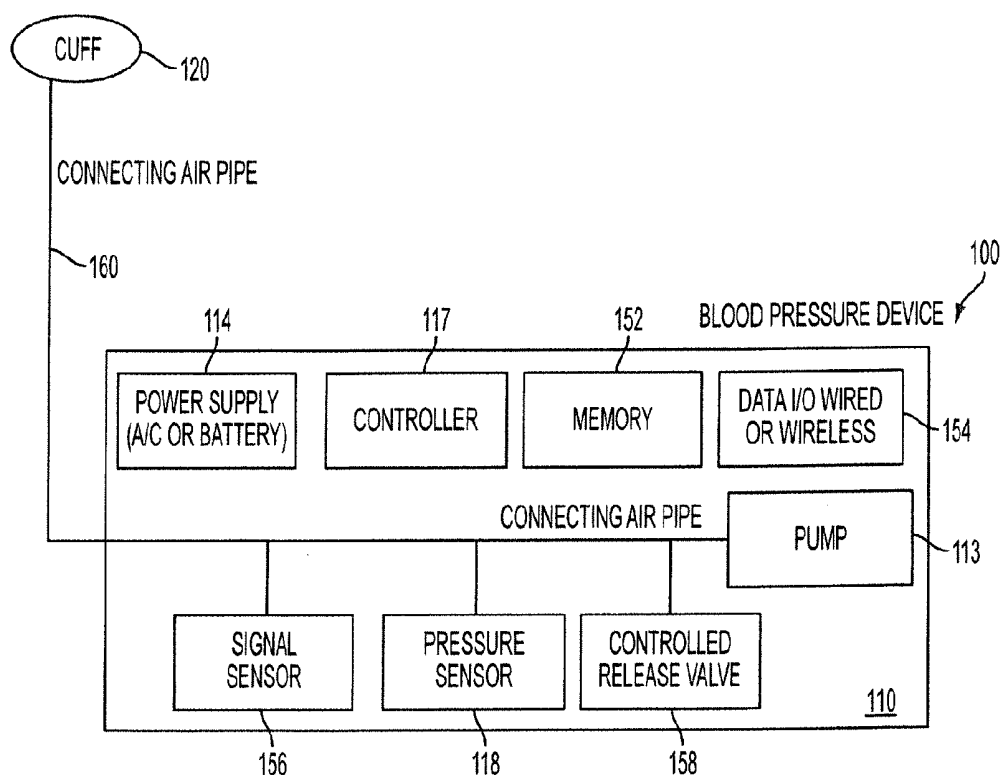
FIG. 1G
