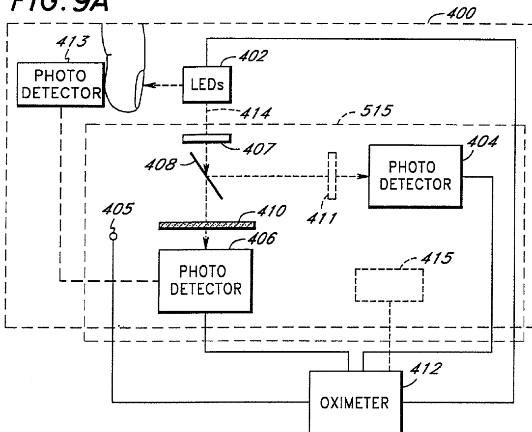
FIG. 9A
