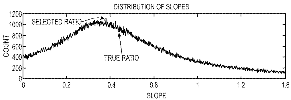
FIG. 7B
