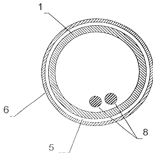
Section 2-2 Fig. 4
