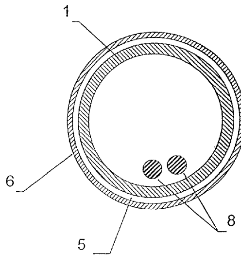
Section 2-2 Fig. 4
