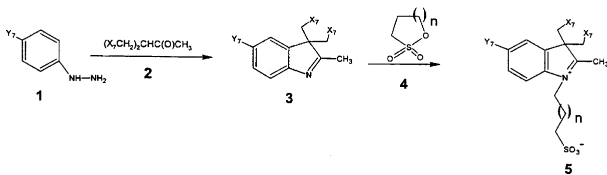
Figure 1: n = 1-3 ; X_7 = H, OH ; Y_7 = H, SO_3^-, CO_2H, CH_2CO_2H, CH_2OH
