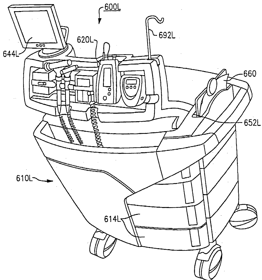
FIG. 41B
