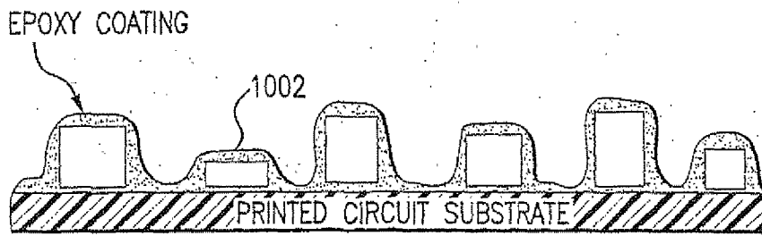
FIG.10B
