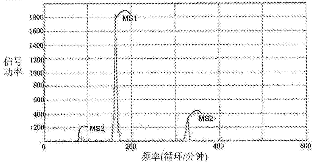
运动传感器功率谱
