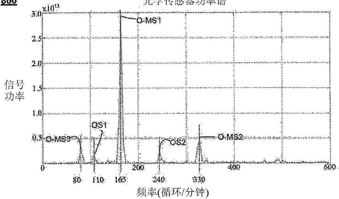
光学传感器功率谱
