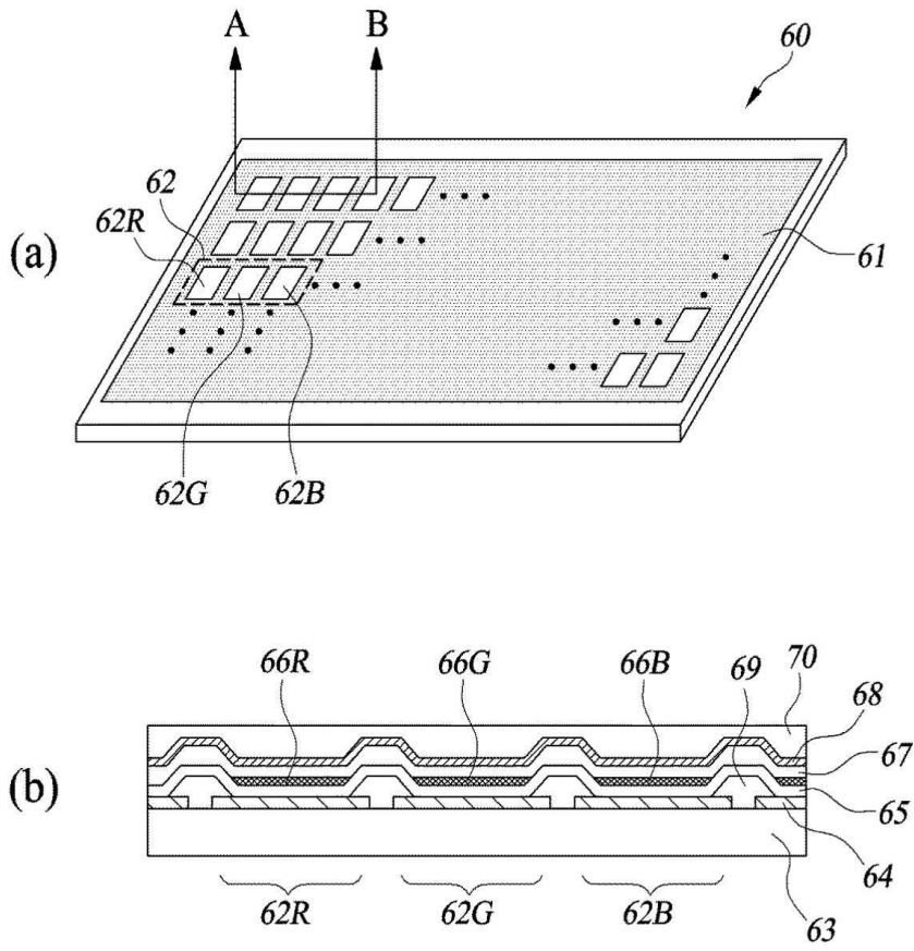
도면7
