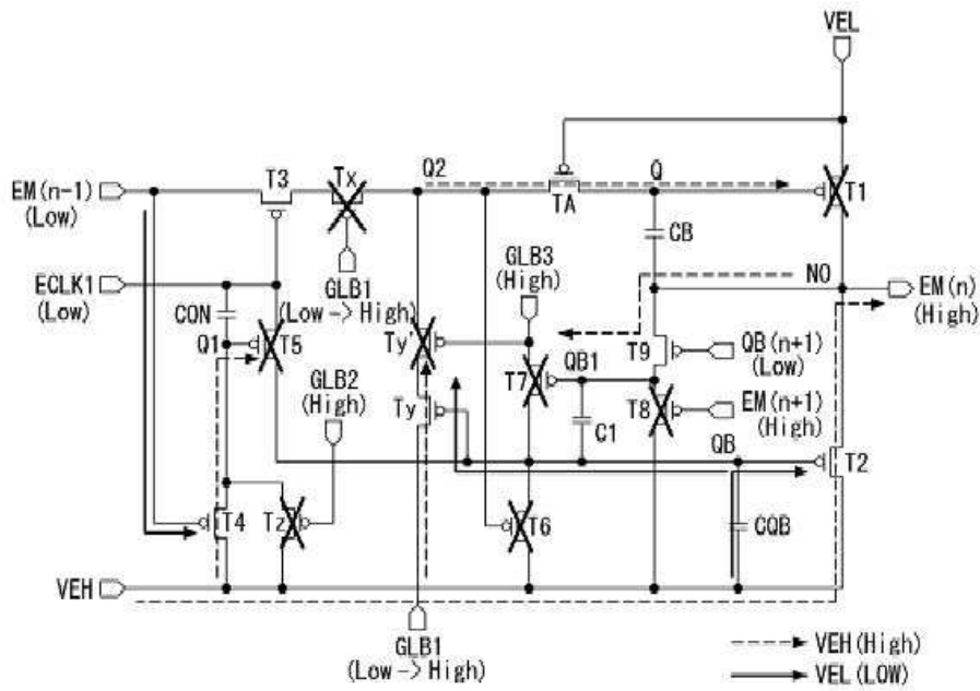
도면12b
