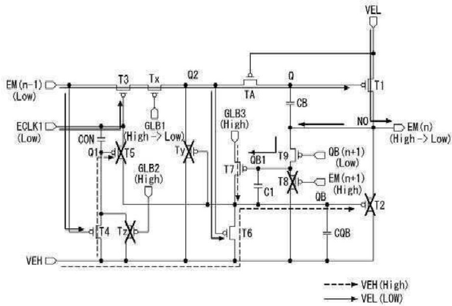
도면9e
