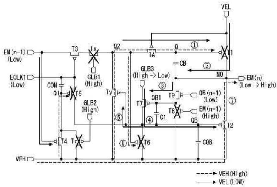
도면9d
