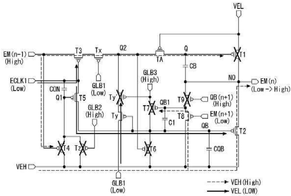
도면12a
