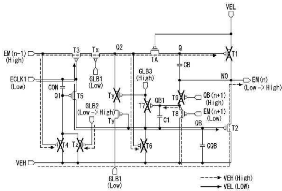
도면12g
