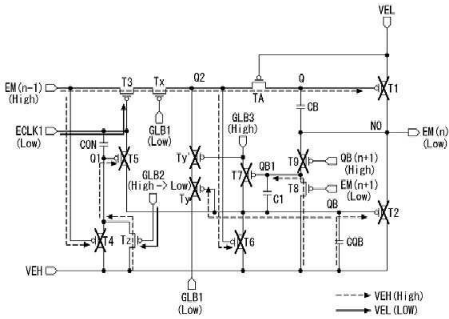
도면12f
