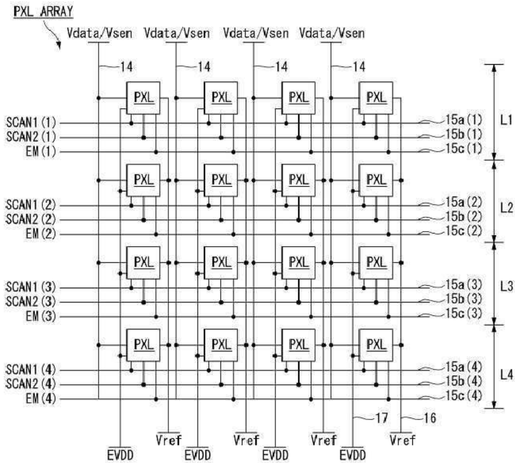
도면3
