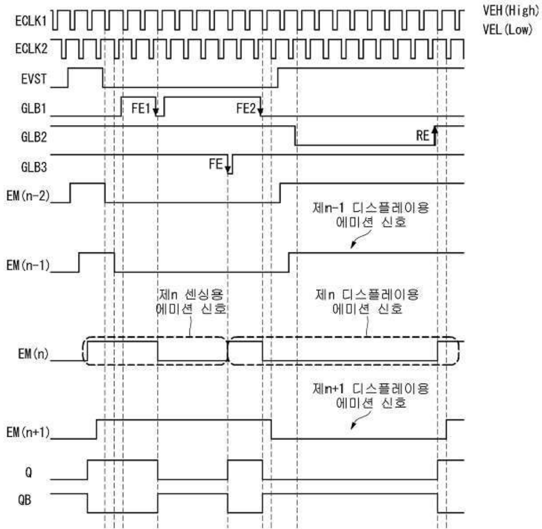
도면11
