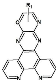
[화학식 11]
