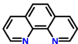
[화학식 13]
