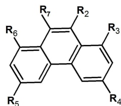
[화학식 11]
