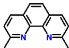
[화학식 14]
